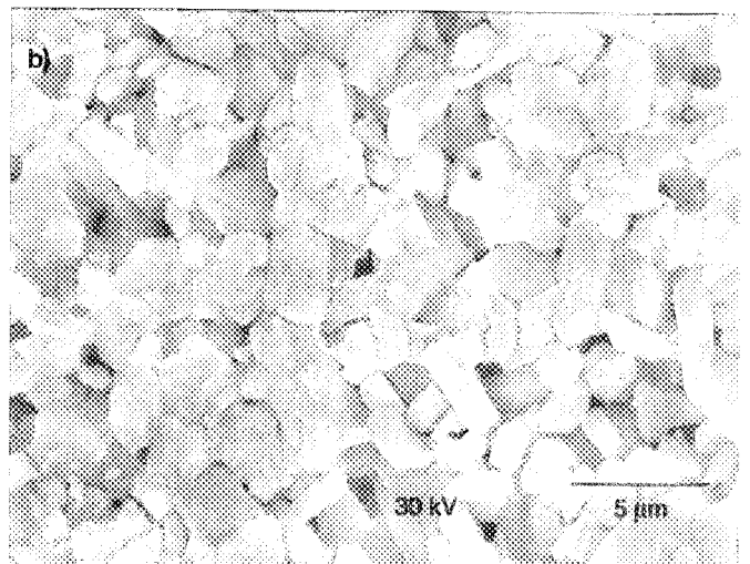
Figura 2. Microestructura de la ferrita de estroncio a 5000 X con x=0 (a) calcinada, (b) sinterizada.
