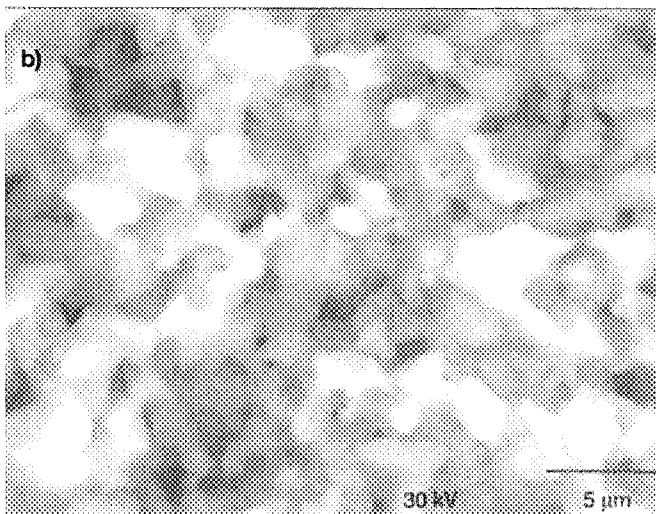
Figura 3. Microestructura de la ferrita de estroncio a 5000 X con x=0.10 (a) calcinada, (b) sinterizada.
