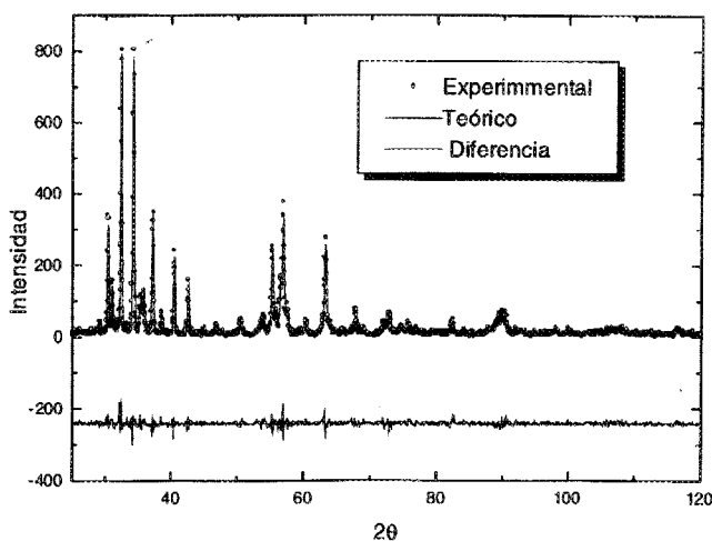
Figura 1. Refinamiento de Rietveld de las ferritas de estroncio (a) x=0 , (b) x=0.10 .
