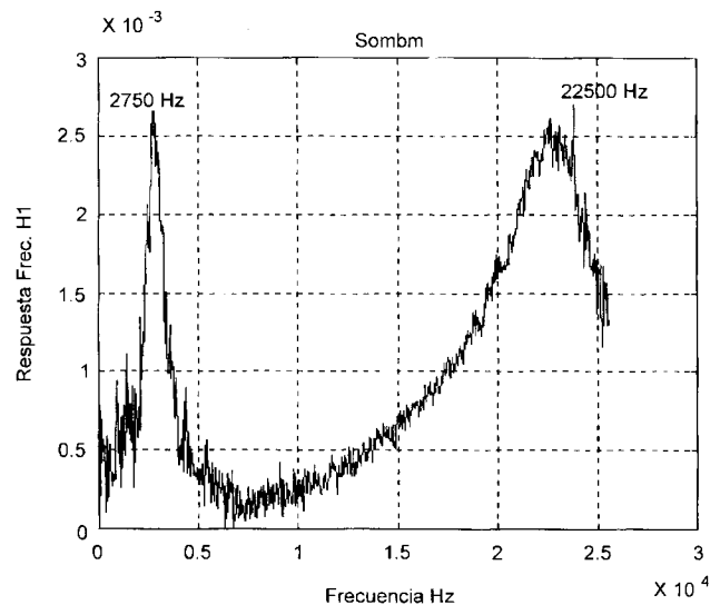
Figura 2. Espectro de resonancia mediante vibrometría láser del cymbal asimétrico (tensión de oscilación de 20 voltios).
