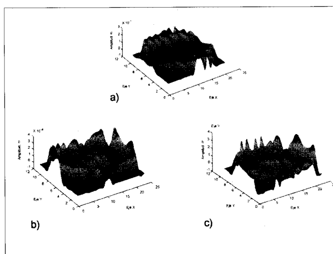
Figura 4. Modos de vibración del címbal asimétrico por la cara del PZT, (a) 2.7 kHz, (b) 8.0 kHz y (c) 11.8 kHz.
