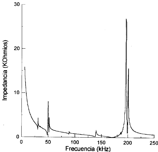
Figura 1. Espectro de resonancia mediante analizador vectorial de impedancias del cymbal asimétrico (tensión de oscilación de 1 voltio).
